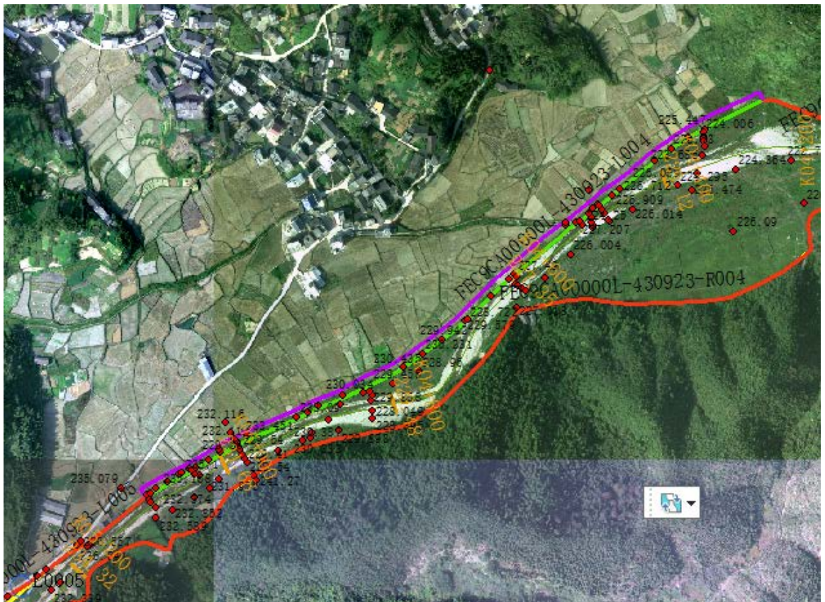
堤脚线外延 10 米划定
