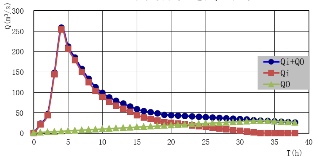
大尧溪十年一遇洪水过程线
