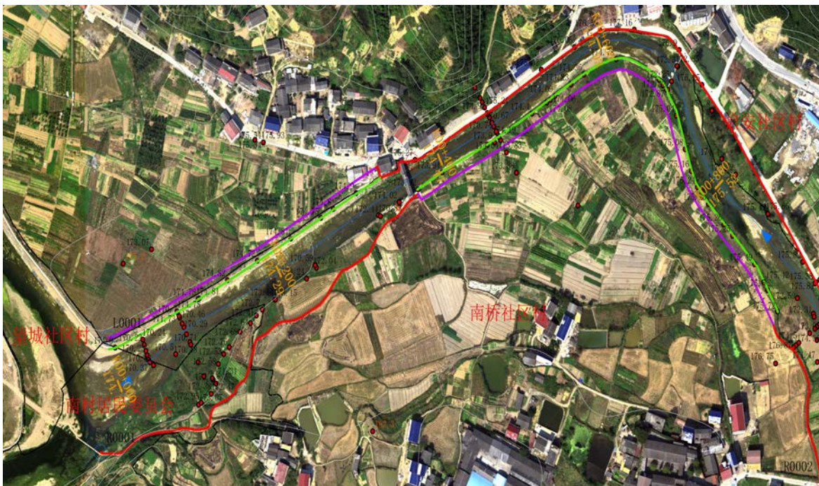
堤脚线外延 10 米划定
