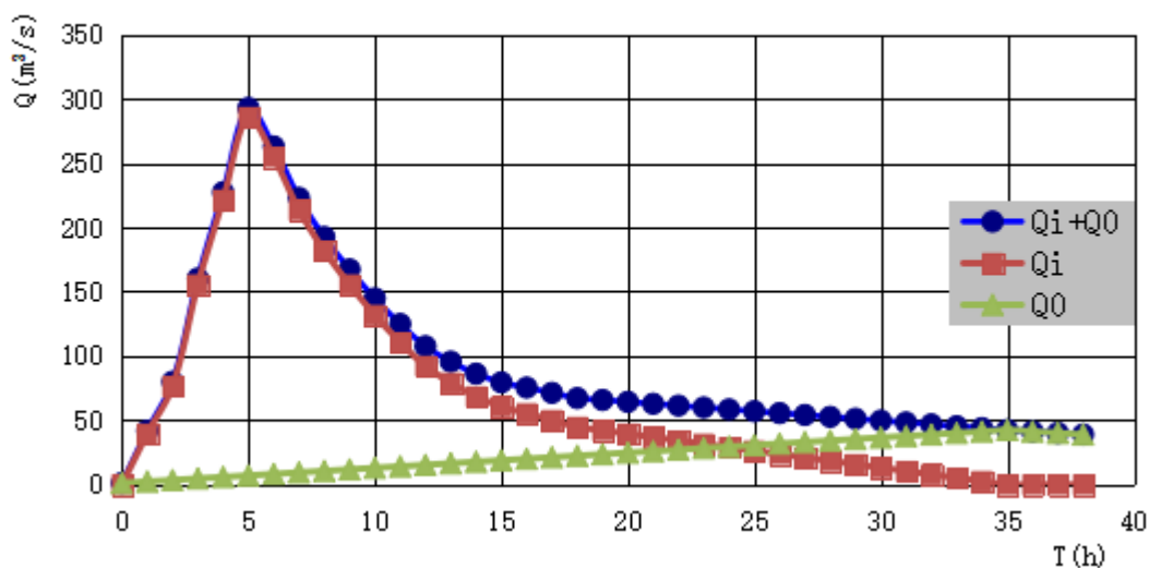
道观坪溪十年一遇洪水过程线
