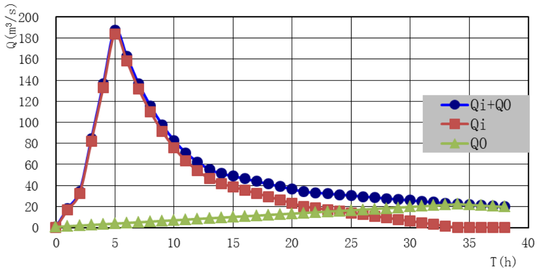
马路溪十年一遇洪水过程线
