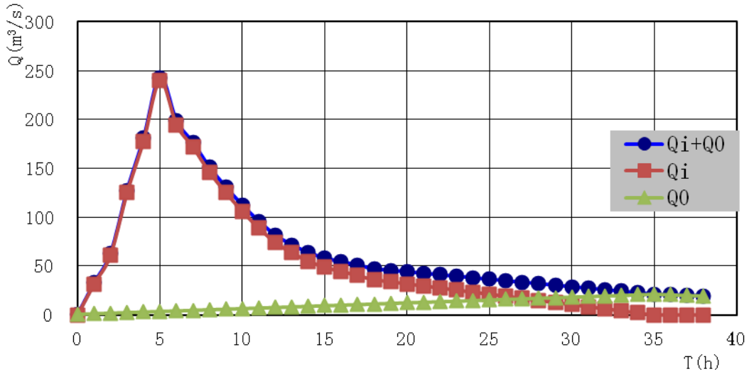
椰子河十年一遇洪水过程线
